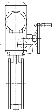
1170-7 mit Elektroantrieb/avec actionneur électrique/with electric actuator
