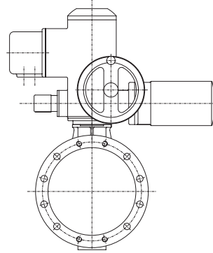
1170-7 mit Elektroantrieb/avec actionneur électrique/with electric actuator
