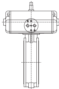
1170-6 mit Pneumatiktrieb/avec actionneur pneumatique/with pneumatic actuator
