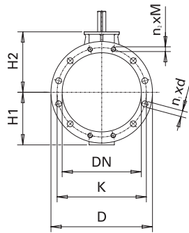
1170-4 mit Getriebe/avec réducteur/with worm gear
